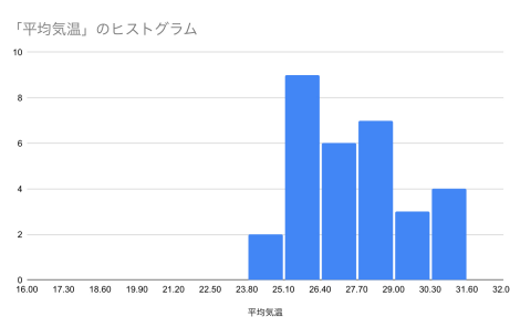
図2：7月の平均気温分布のヒストグラム
