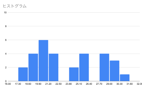
図1：6月の平均気温分布のヒストグラム
